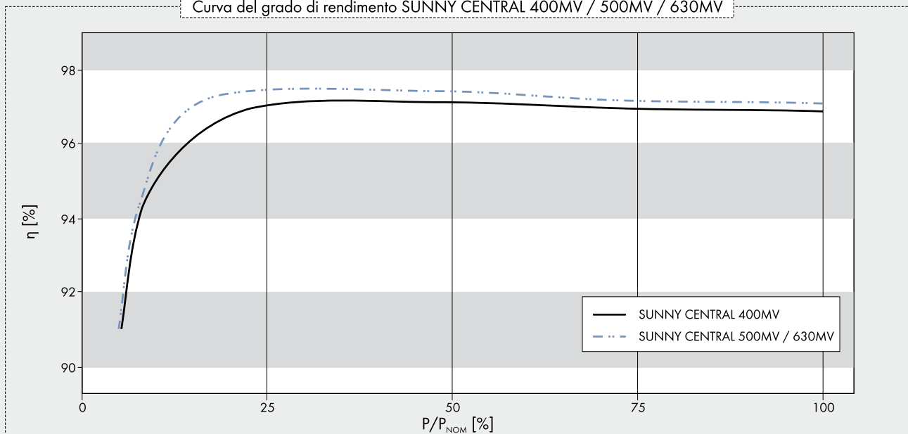
Curva del grado di rendimento SUNNY CENTRAL 400MV / 500MV / 630MV
