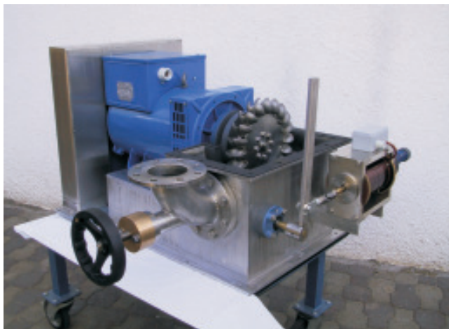
Turbine tipo Pelton con generatore sincrono 15 KVA - 1500 g/min. - 150m dislivello
