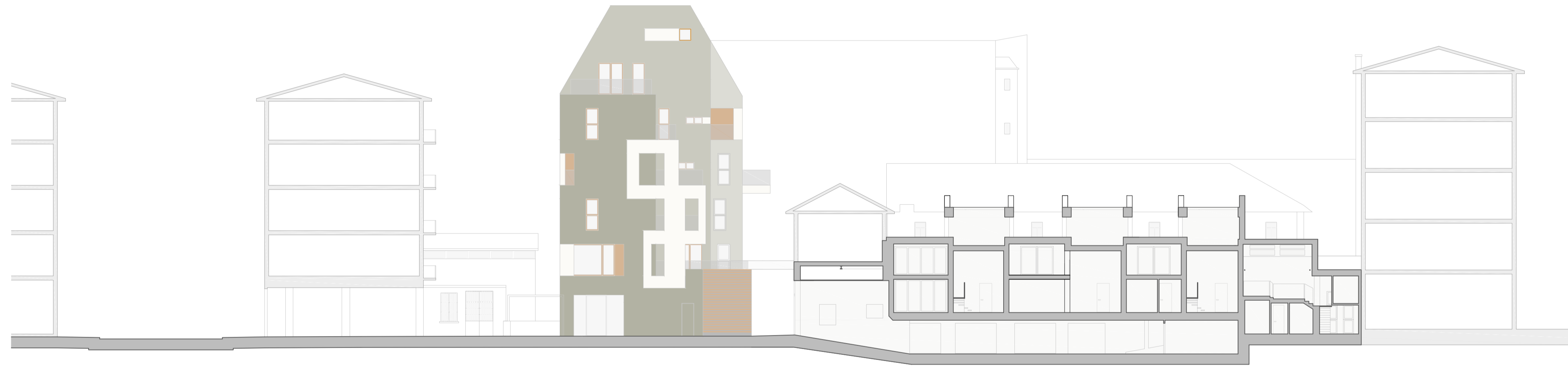
K19A+B - sezione attraverso l'isolato
