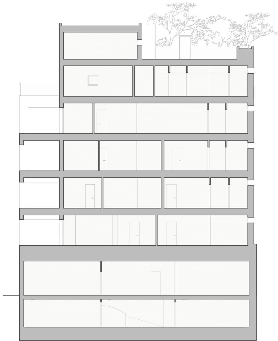
K19B - sezione BB
