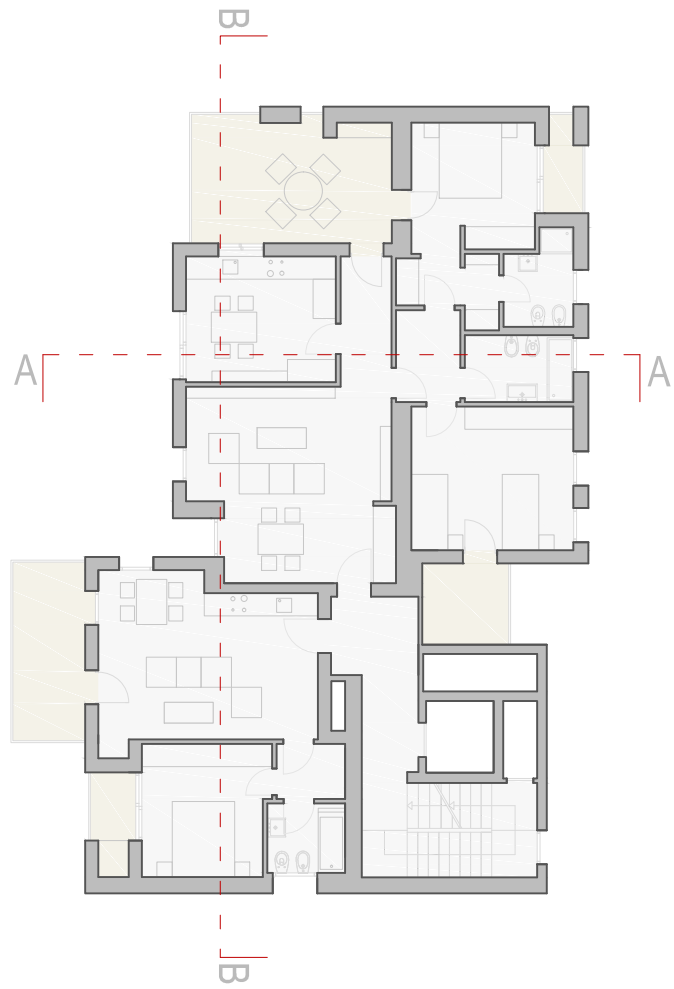
K19B - pianta piano terzo
