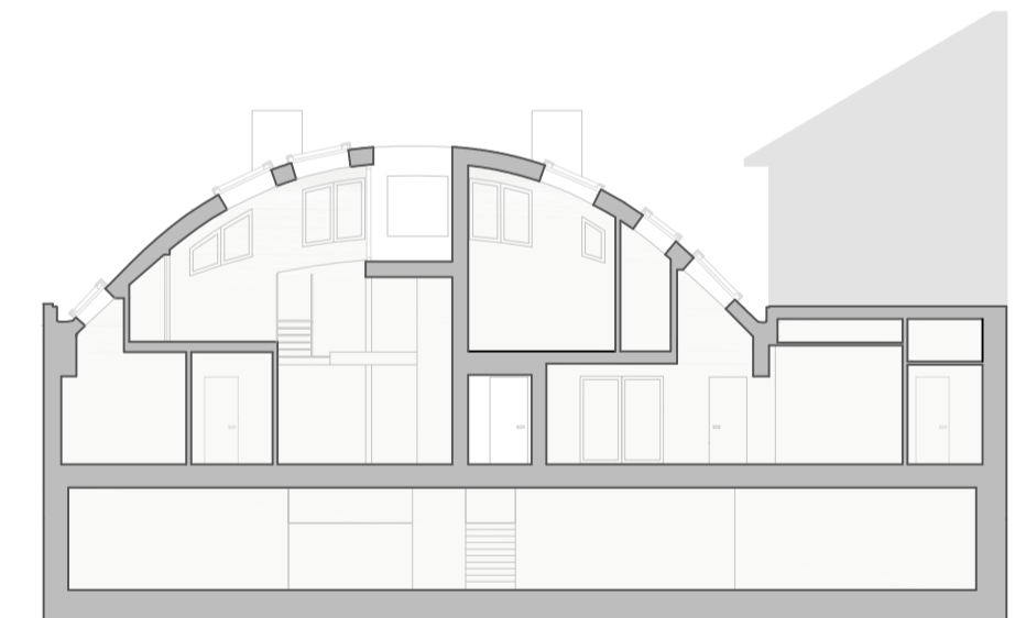
K19A - sezione FF
