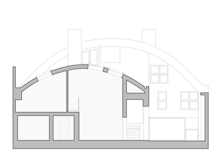
K19A - sezione EE
