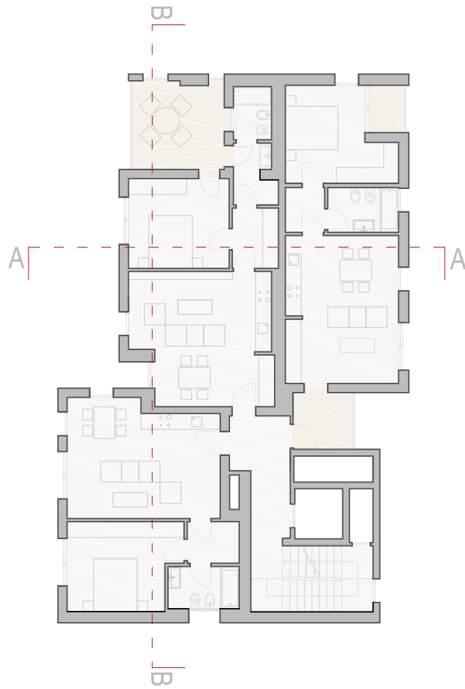
K19B - pianta piano secondo
