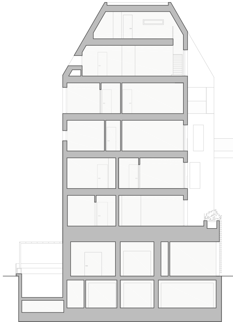
K19B - sezione AA
