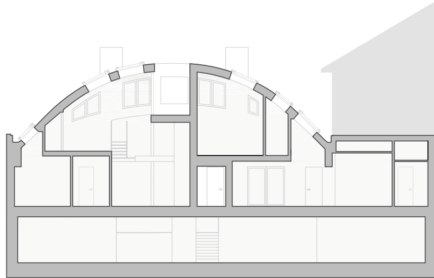
K19A - sezione FF
