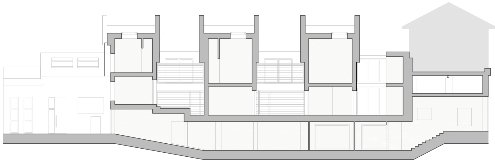
K19A - sezione DD
