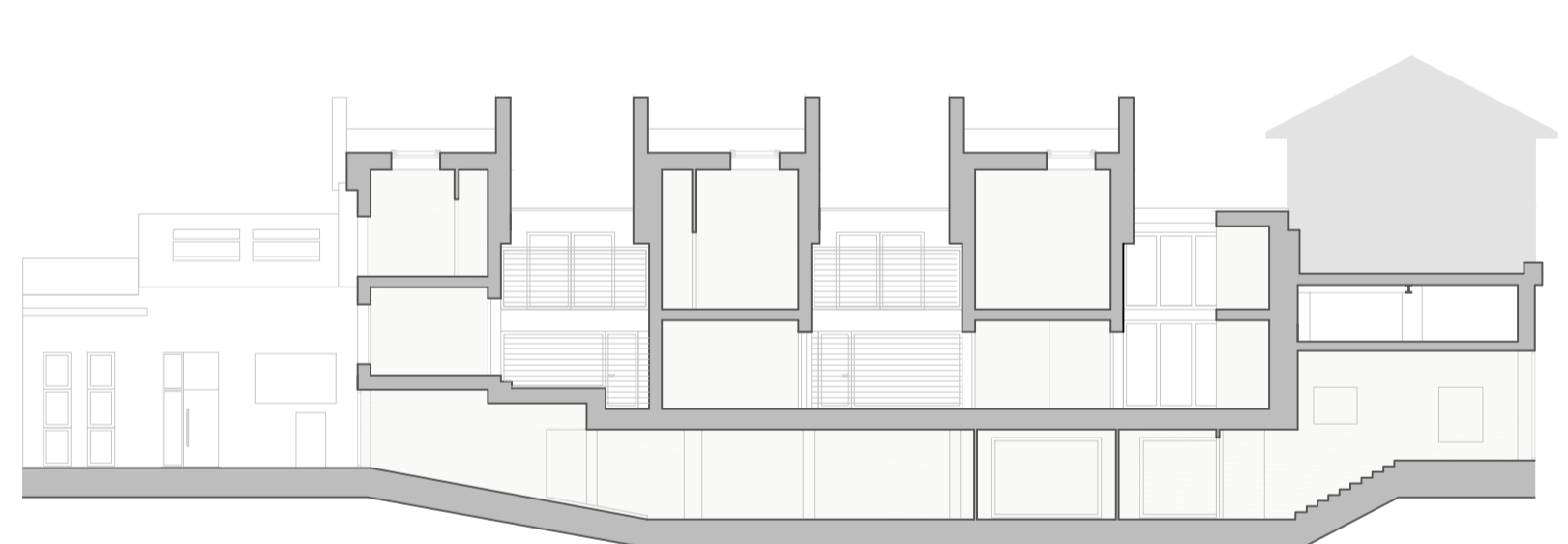
K19A - sezione DD
