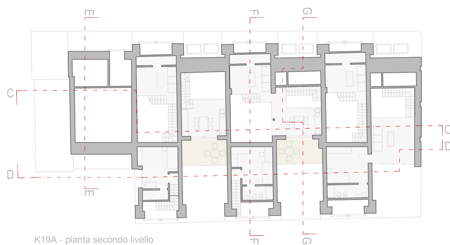
K19A - pianta secondo livello
