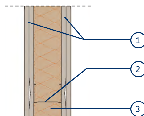
1. Lastre di gesso rivestito 2. Struttura in acciaio zincato
