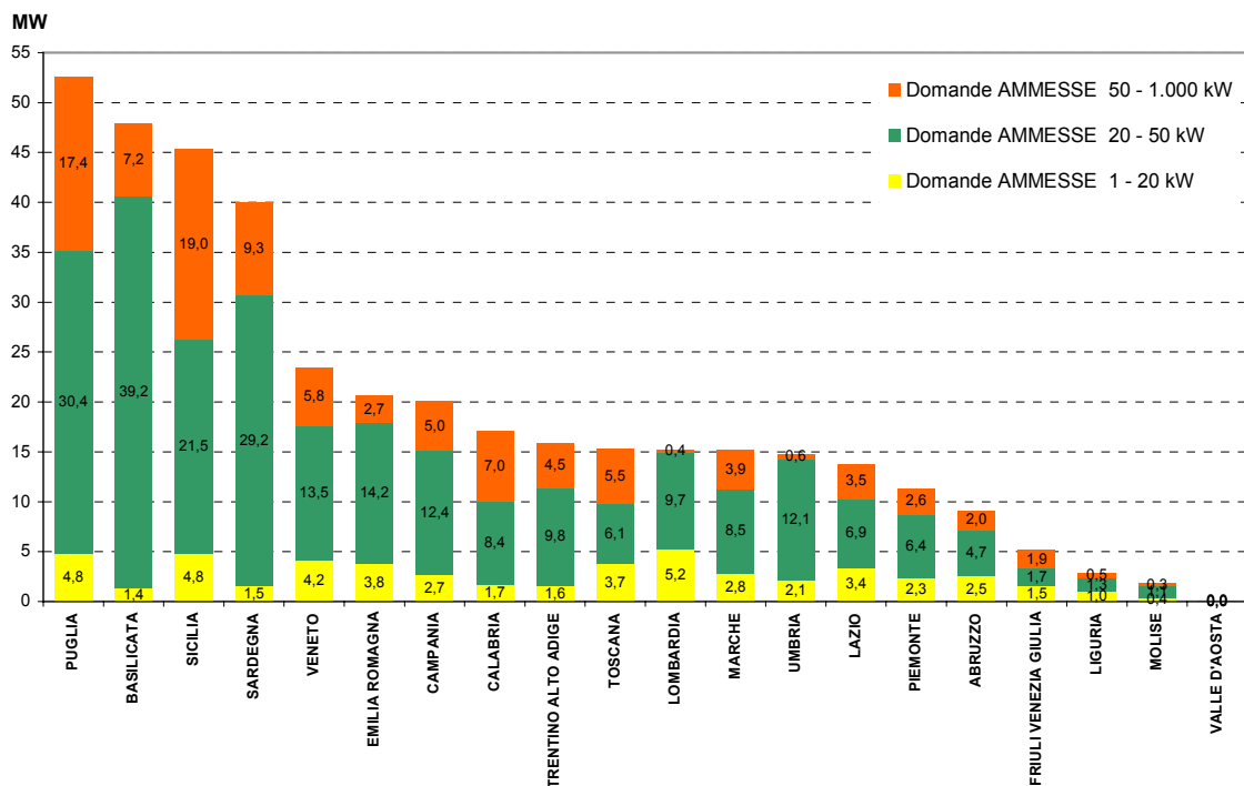
Fig. 5 – ripartizione del numero delle domande ammesse per regione
