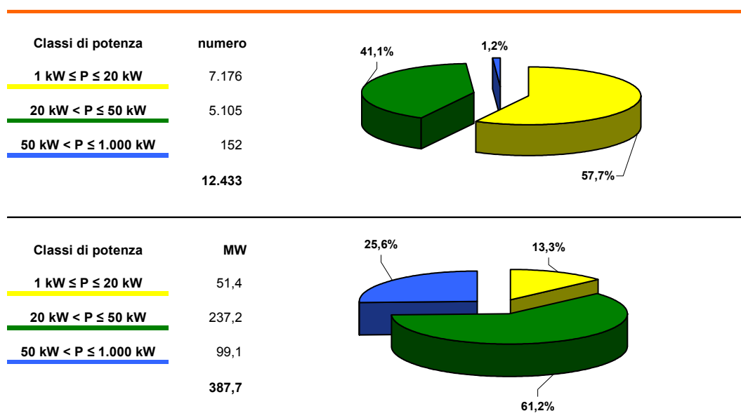
Fig. 3 - ripartizione delle domande ammesse ad incentivazione
