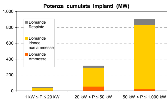
Potenza (MW) domande ammesse: ripartizione tra le tre classi di potenza
