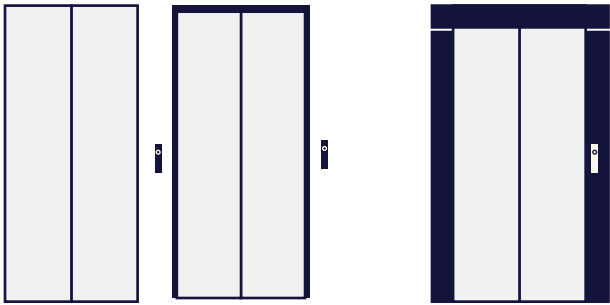
Senza telaio Telaio ridotto Spessore 20 mm Spessore 150 mm: standard Spessore 100 mm: optional
