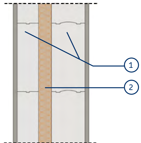
1. Pareti in blocchi di calcestruzzo 2. URSA TERRA 66 cellulare autoclavato
