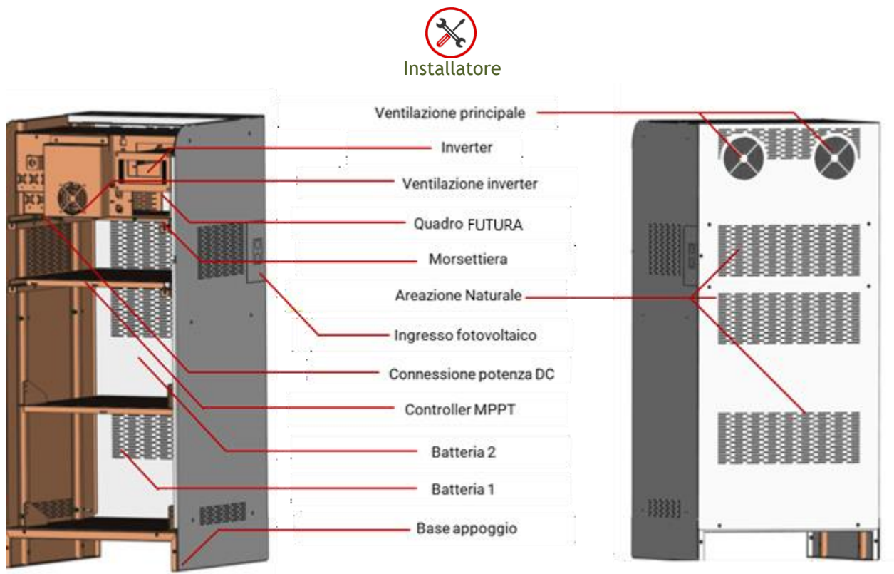
Figura 6- Distribuzione componenti FUTURA
