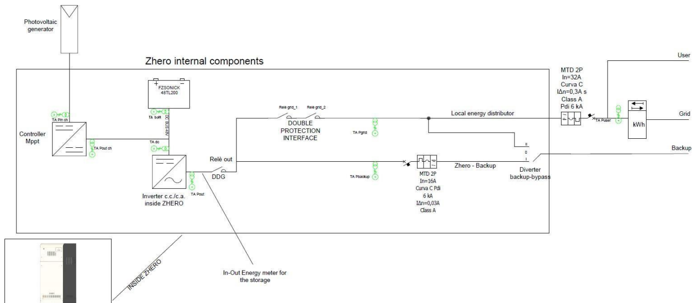
Figura 5- Schema a Blocchi FUTURA
