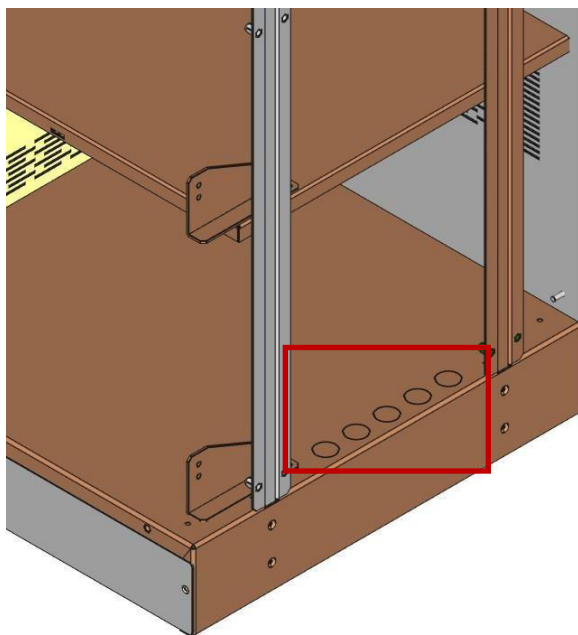
Figura 13 - Dettaglio spacchi FUTURA
