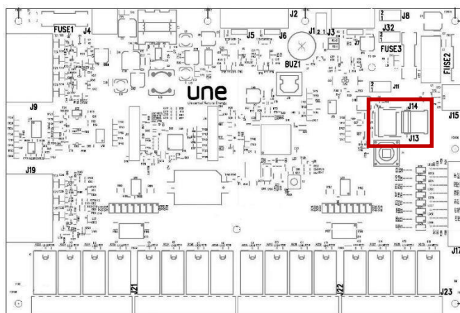
Figura 74 - Posizione della micro SD nella scheda CPU
