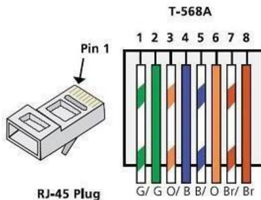
Figura 18 - Pin collegamento del connettore RJ-45
