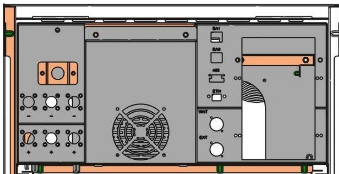
Figura 19- Dettaglio connessione wattmetro
