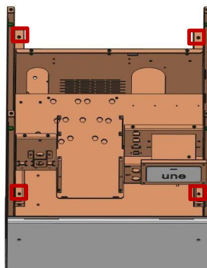
Figura 73 - Posizione delle viti di fissaggio del cassetto
