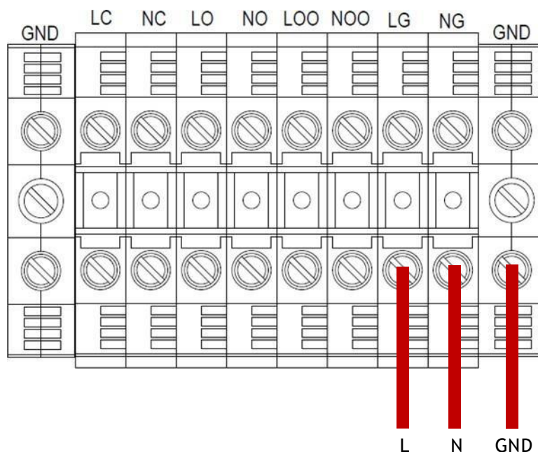
Figura 15 - Morsettiera collegamento
