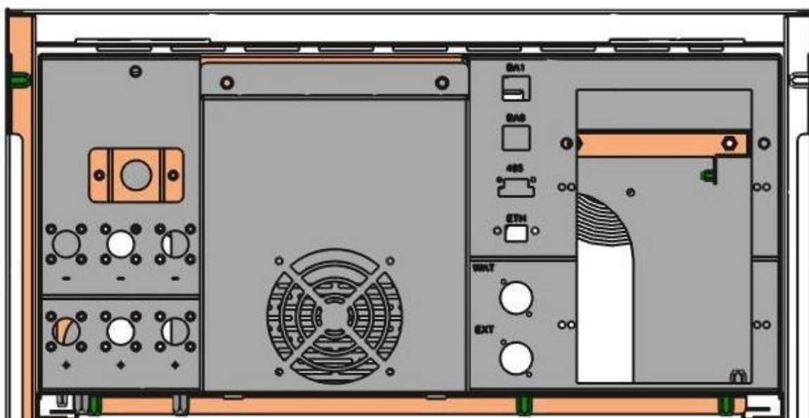
Figura21-Dettaglioconnessioneethernet
