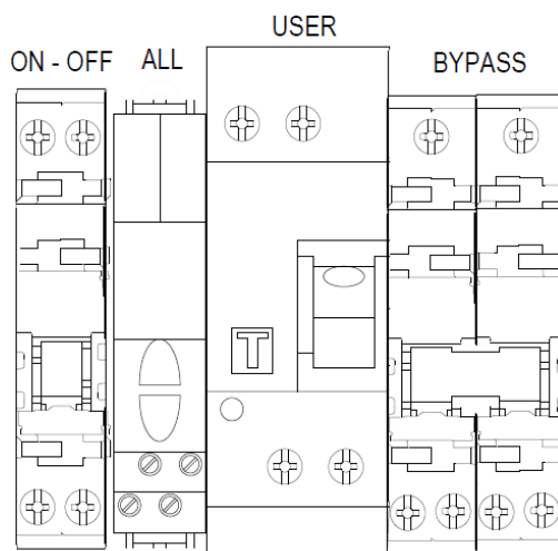
Figura 22- Quadro FUTURA
