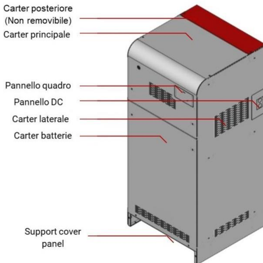
Figura 66 - Nomi e posizione dei carter del sistema
