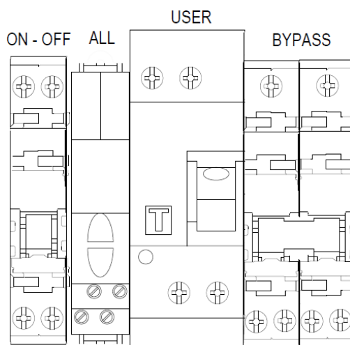
Figura 4 - Quadro FUTURA
