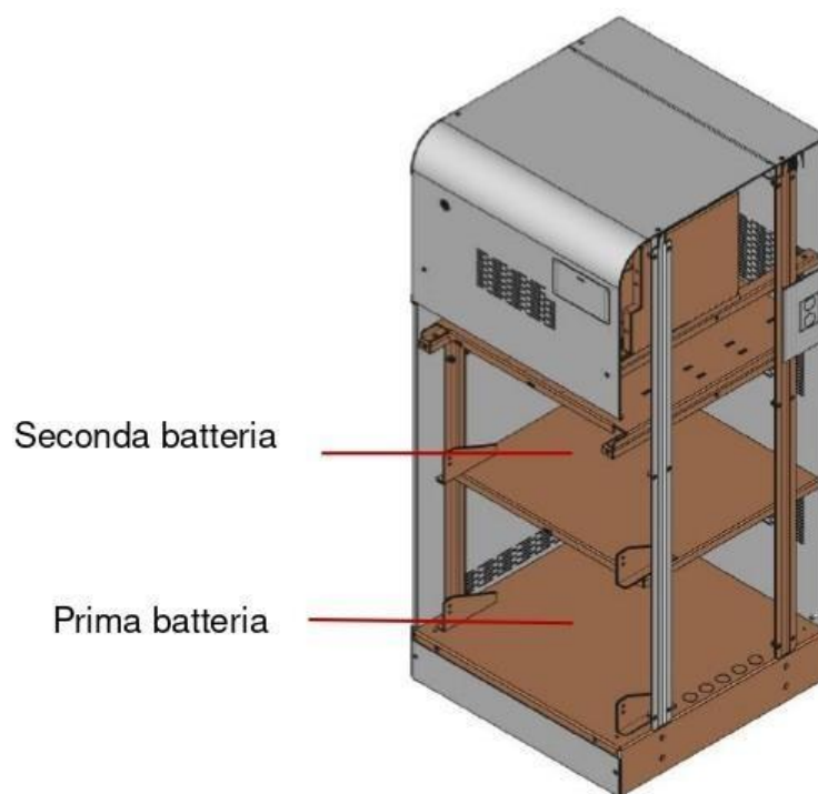
Figura 10 - FUTURA
