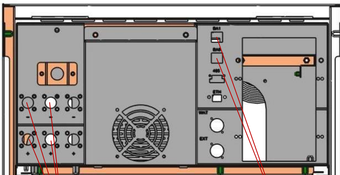
Figura 12- Cassettoinverter FUTURA
