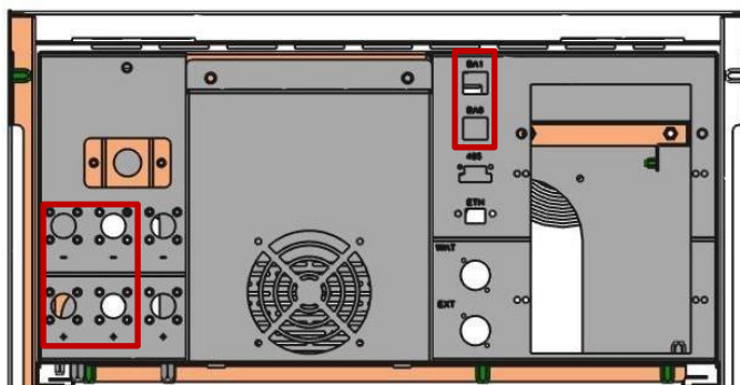
Figura 67 - Posizione dei plug batteria e delle connessioni con RJ-45
