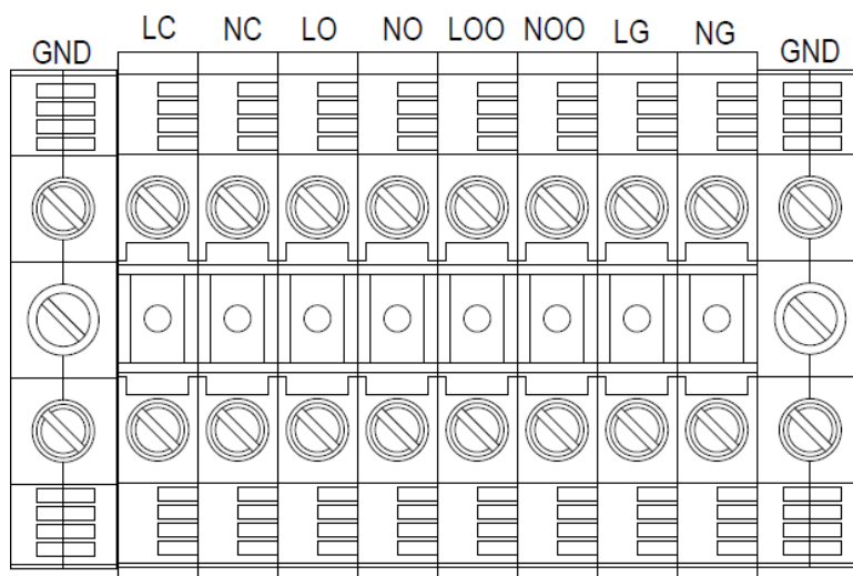
Figura 14 - Morsettiera lato AC
