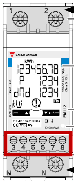
Figura 20 - Morsettiera collegamento al wattmetro
