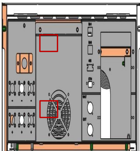
Figura 68 - Posizione delle staffe di ancoraggio della batteria
