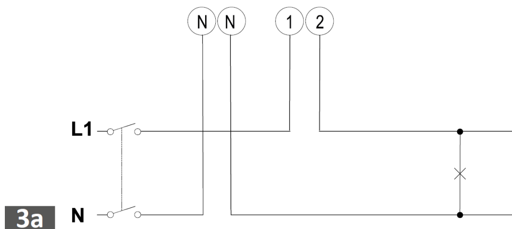
Figura 17 - Collegamento linea elettrica sul wattmetro
