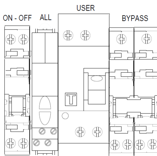
Figura 61 - Quadro FUTURA
