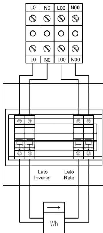
Figura 16 - Schema esemplificativo “entra-esce” contatore
