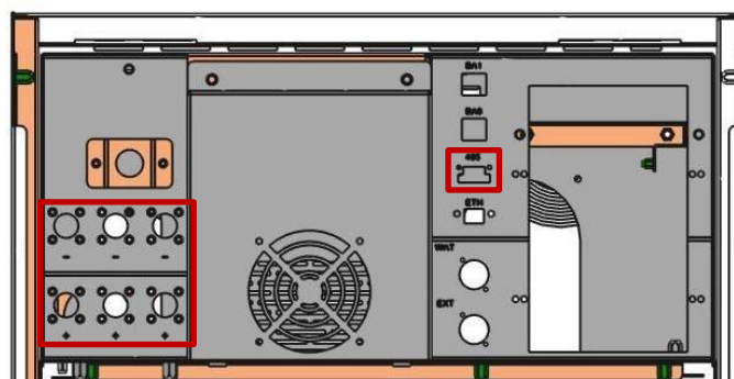
Figura 70 - Connettore 485 e posizione dei plug di potenza
