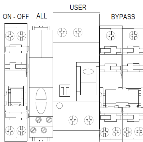
Figura 7 - Rappresentazione quadro FUTURA
