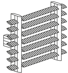
D1 - Frangisole orizzontale. Angoli prestabiliti e variabili. Collegabile alle facciate continue METRA Building ed alla muratura. D1 - Horizontal sunblades. Angles are preset and variable. Can be connected to the METRA Building curtain walls and to the wall.
