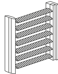
D3 - Frangisole orizzontale. Angoli prestabiliti e variabili. Collegabile frontalmente e lateralmente alla muratura ed alle sottostrutture in acciaio. D3 - Horizontal sunblades. Angles are preset and variable. Can be connected frontally and laterally to the wall and to the steel substructure.
