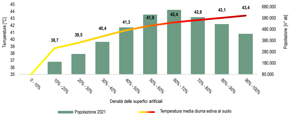
Figura 154. Andamento della temperatura media diurna estiva al suolo (LST) (°C) per gli anni dal 2019 al 2024 e numero di abitanti (2021) esposti per classi di densità delle superfici artificiali
